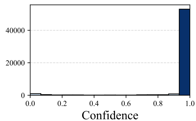
Llama-4-Scout-17B-16E-Instruct
