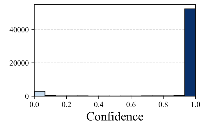
gemma-3-27b-it
