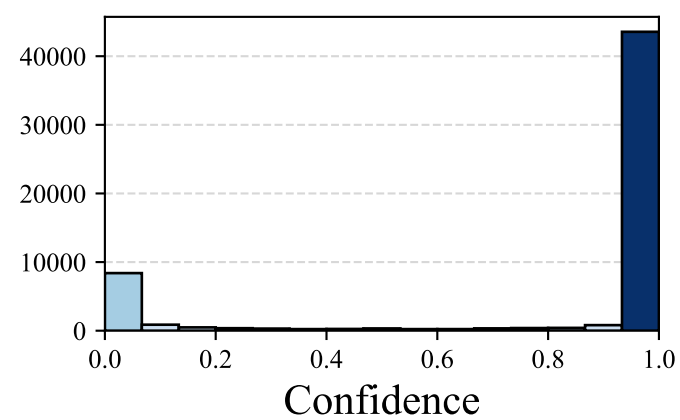
Llama-3.3-70B-Instruct
