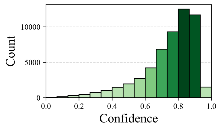
Qwen3-30B-A3B-Thinking-2507
