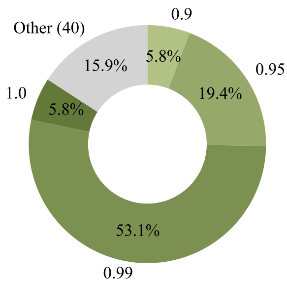
gpt-oss-20b
