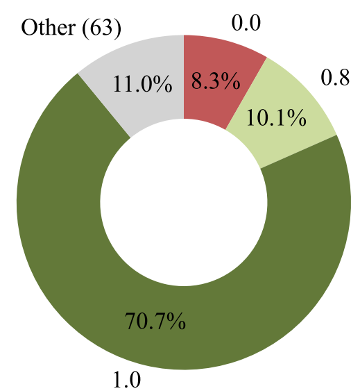
Llama-4-Scout-17B
