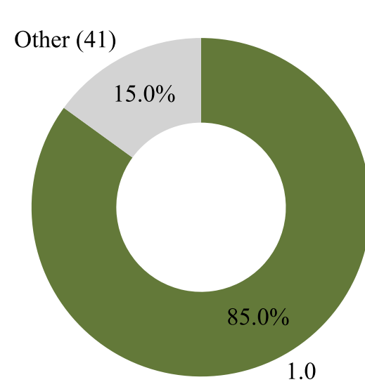
Qwen3-30B-A3B-Thinking
