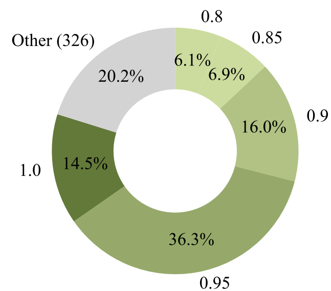
DeepSeek-Qwen-32B
