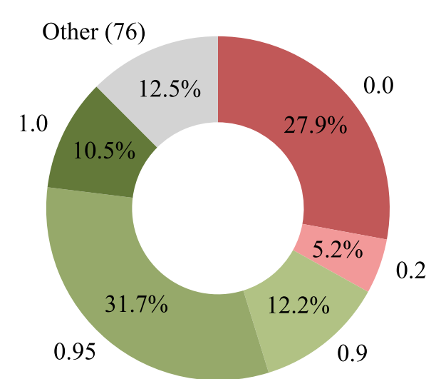
Mistral-Nemo-7B
