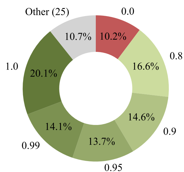
Llama-3.3-70B
