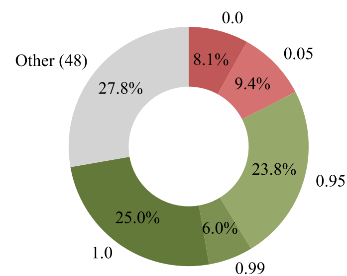
google/gemma-3-27b
