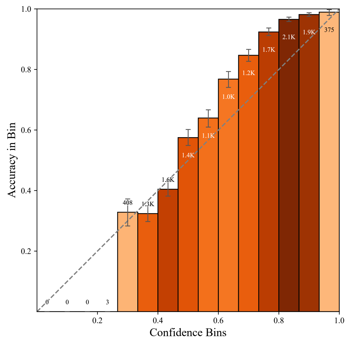
MMLU
