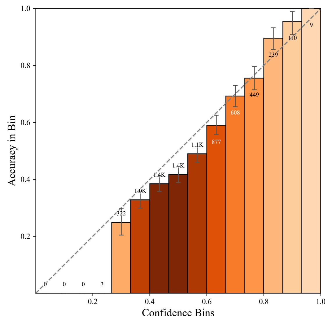
GSM8KMC
