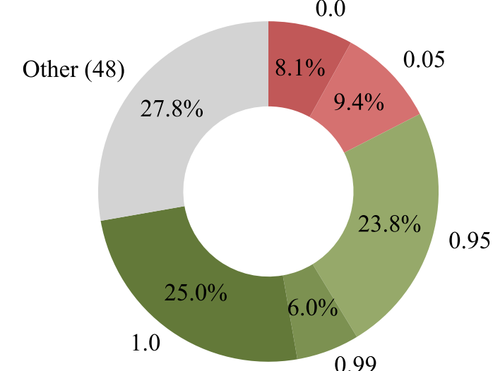
google/gemma-3-27b
