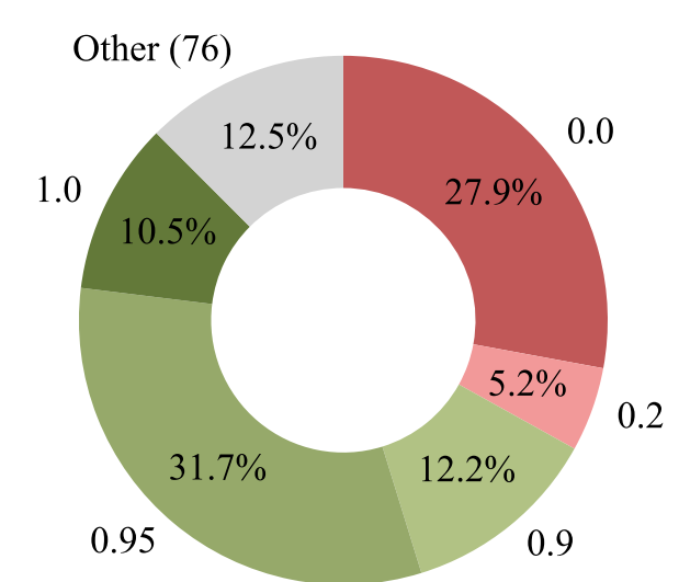
Mistral-Nemo-7B
