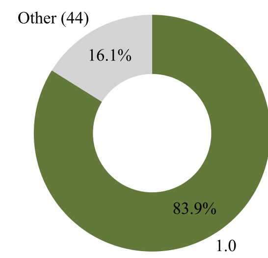
Qwen3-30B-A3B-Thinking
