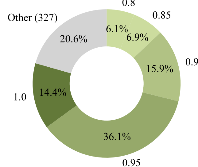
DeepSeek-Qwen-32B
