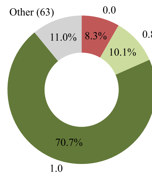
Llama-4-Scout-17B
