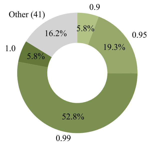
gpt-oss-20b
