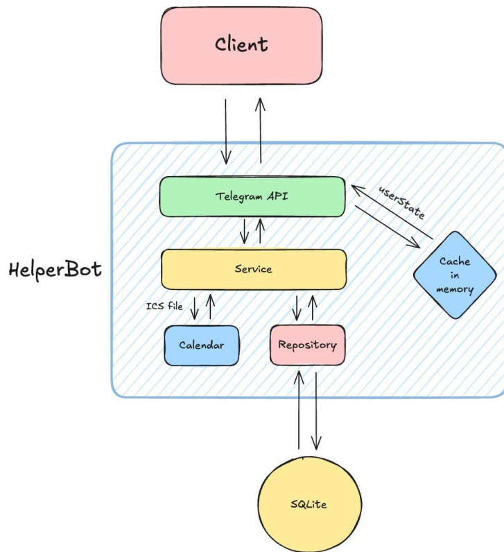
Рисунок 1. Архитектура приложения
