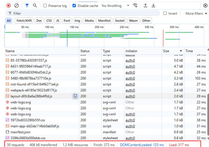
Gambar 4.40 Hasil dari “ Network Monitor ” halaman login
