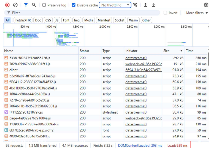
Gambar 4.43 Hasil dari “ Network Monitor ” halaman datastreams
