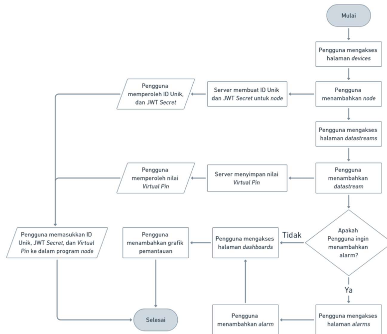
Gambar 3.8 Diagram alur penggunaan antarmuka aplikasi
