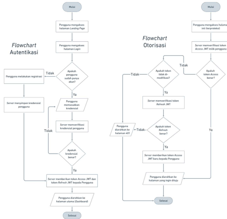
Gambar 3.7 Diagram alur autentikasi dan otorisasi pengguna
