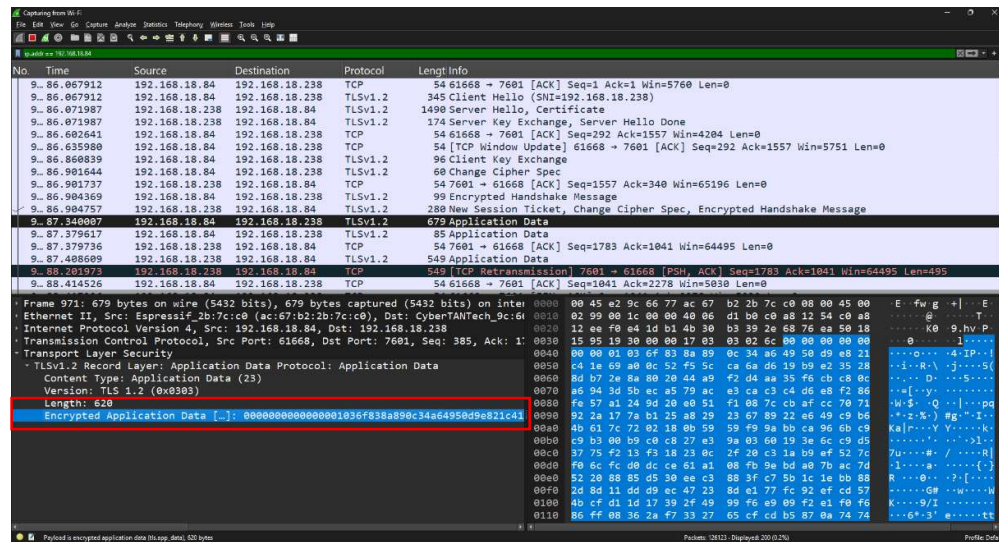
Gambar 4.34 Payload HTTPS pada Aplikasi Wireshark
