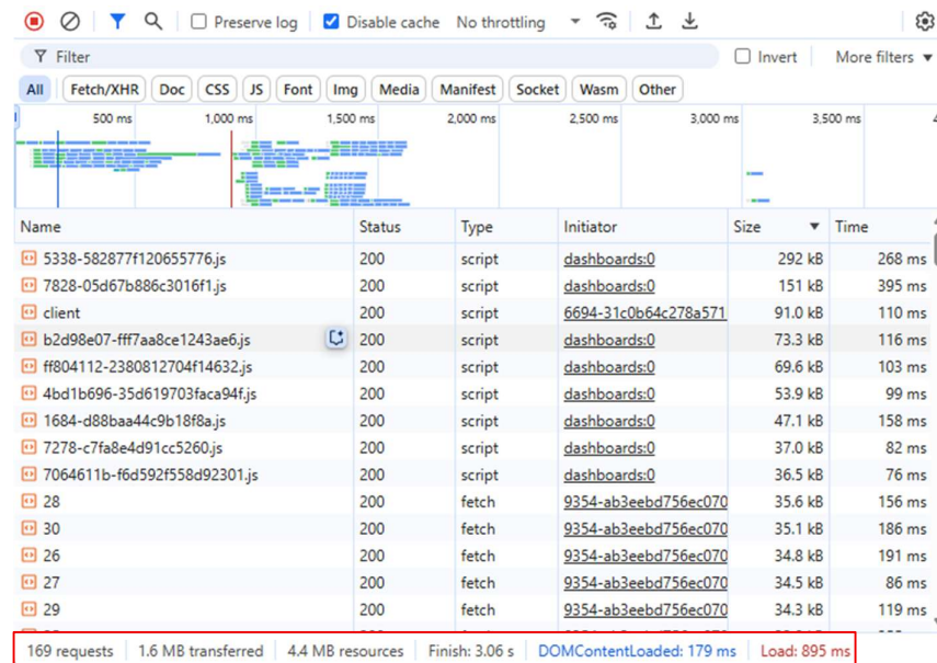
Gambar 4.41 Hasil dari “ Network Monitor ” halaman dashboards
