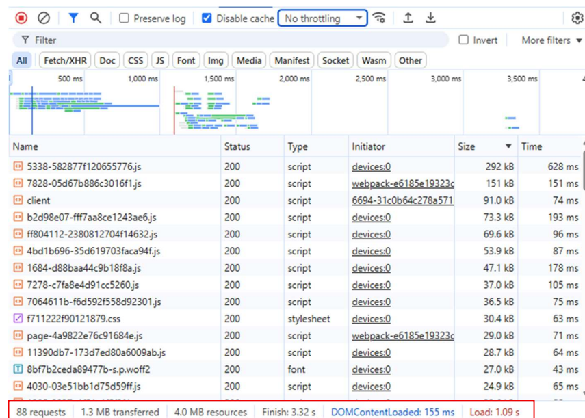
Gambar 4.42 Hasil dari “ Network Monitor ” halaman devices
