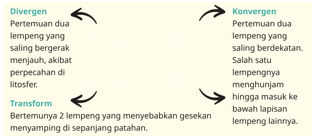
Gambar 3.10 Pergerakan Lempeng Tektonik
