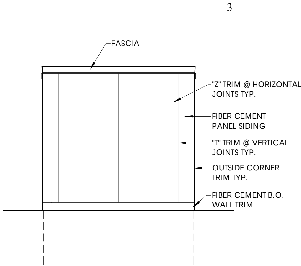
A3 A2.03 PATIO BAR WEST 1/4" = 1'-0"
