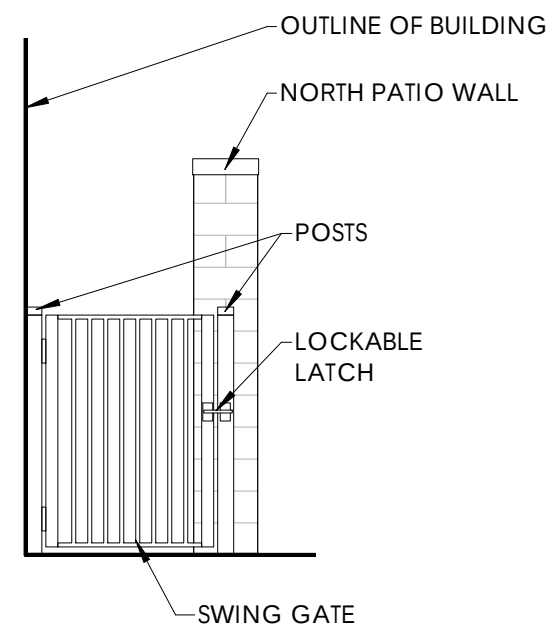
A3 A2.03 PATIO BAR WEST 1/4" = 1'-0"
