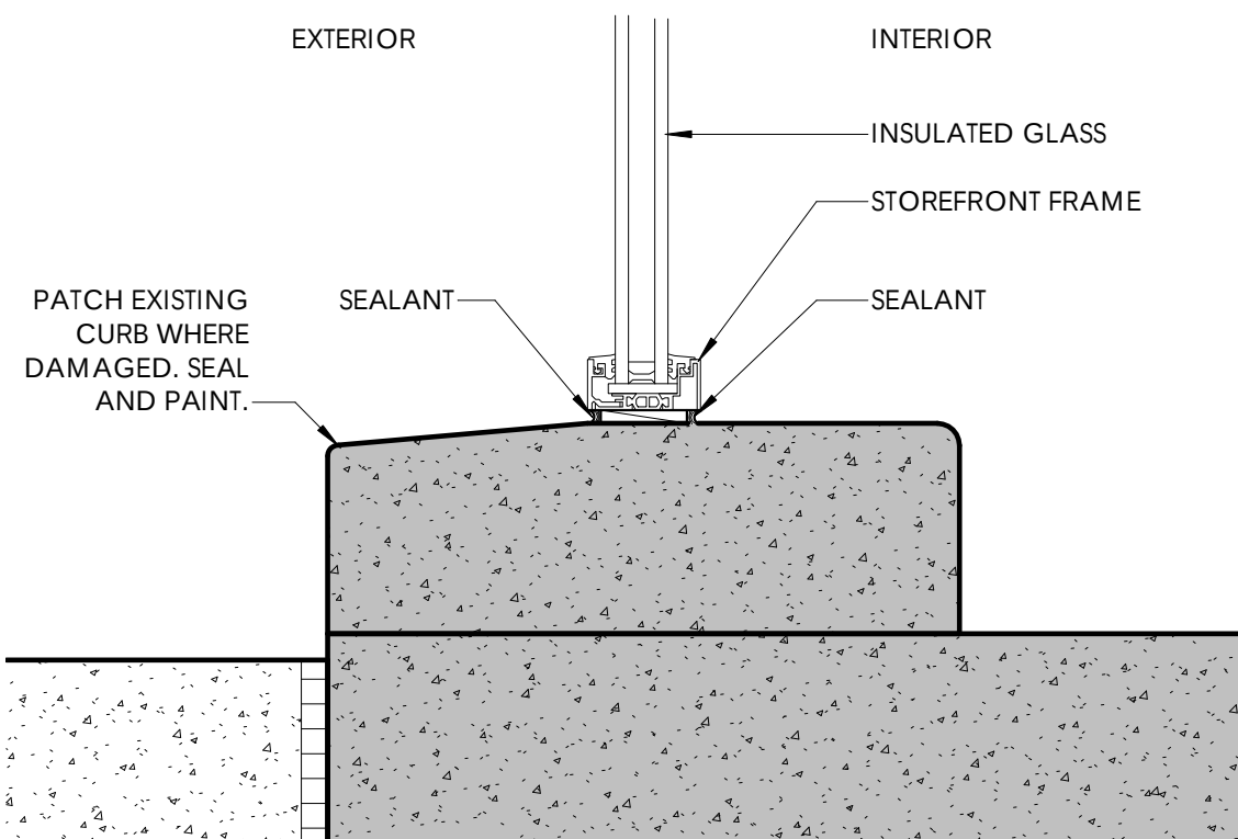
D1 A7.02 LOBBY WINDOW SILL 3" = 1'-0"
