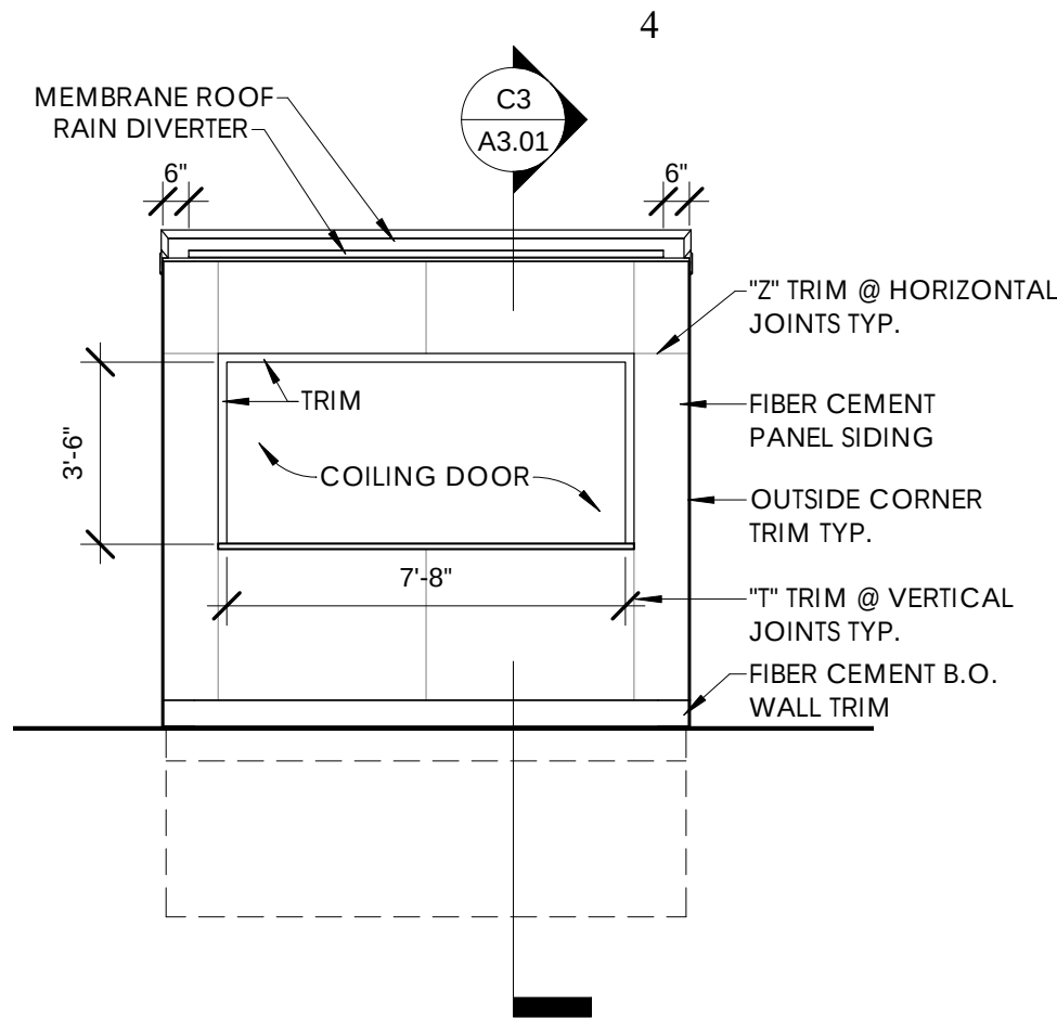
A4 A2.03 PATIO BAR EAST 1/4" = 1'-0"
