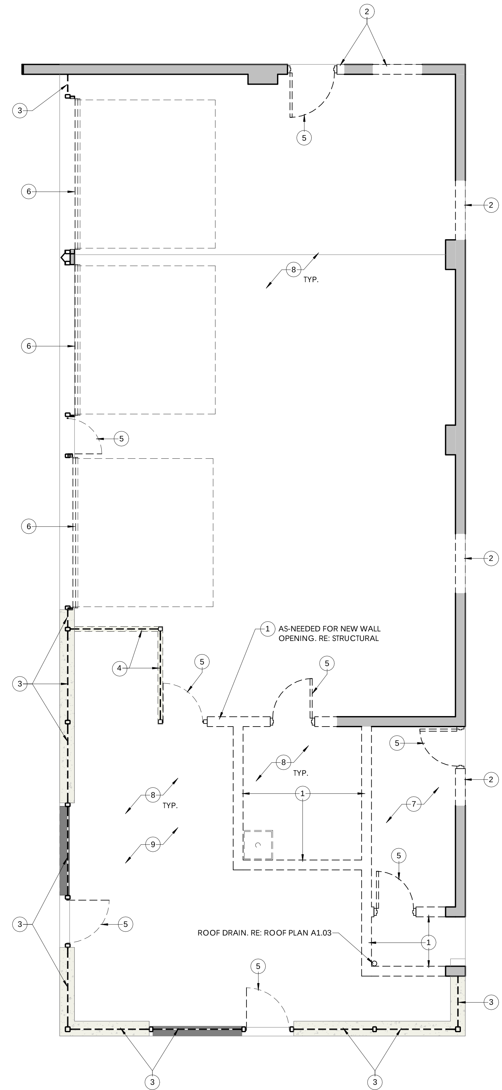
D2 D1.01 DEMOLITION PLAN 1/4" = 1'-0"
