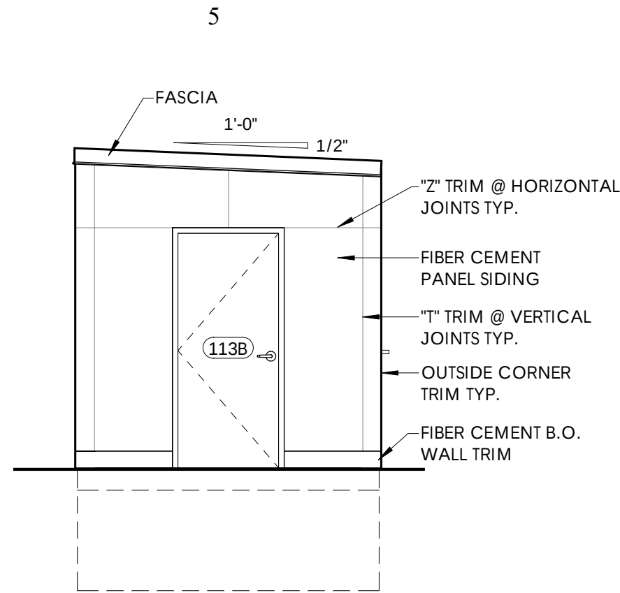
A5 A2.03 PATIO BAR SOUTH 1/4" = 1'-0"
