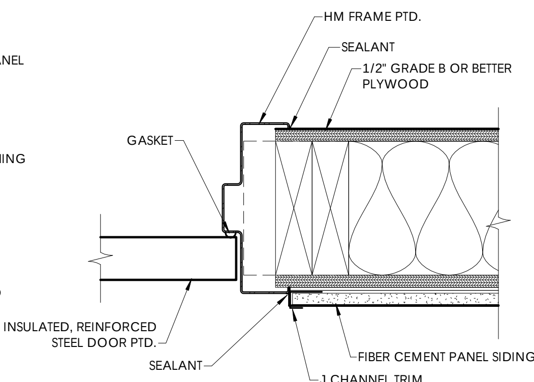
D3 A7.02 PATIO BAR DOOR JAMB 3" = 1'-0"
