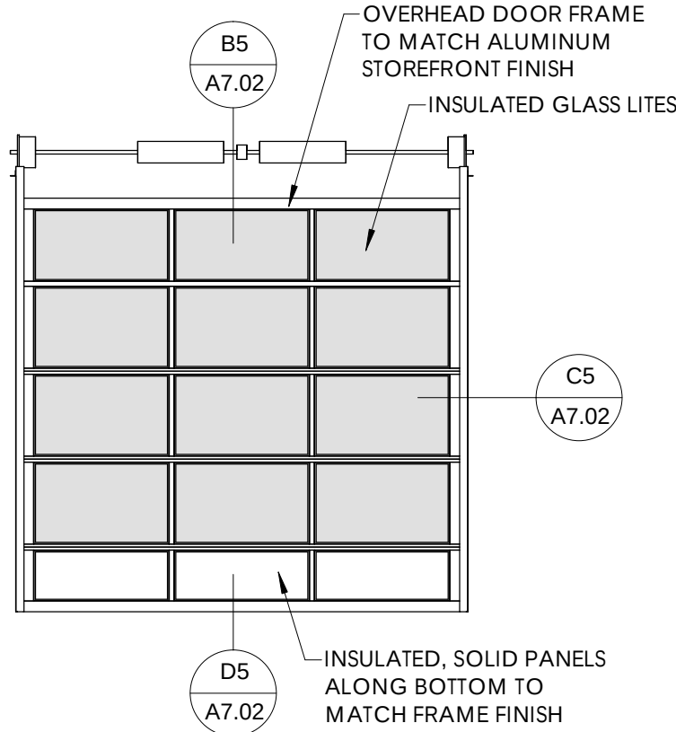
OVERHEAD DOOR
