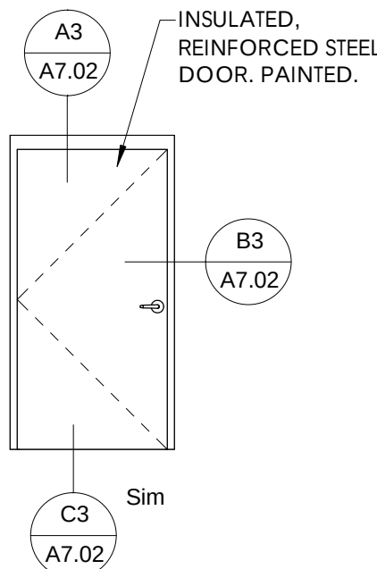
DOOR TYPE B
