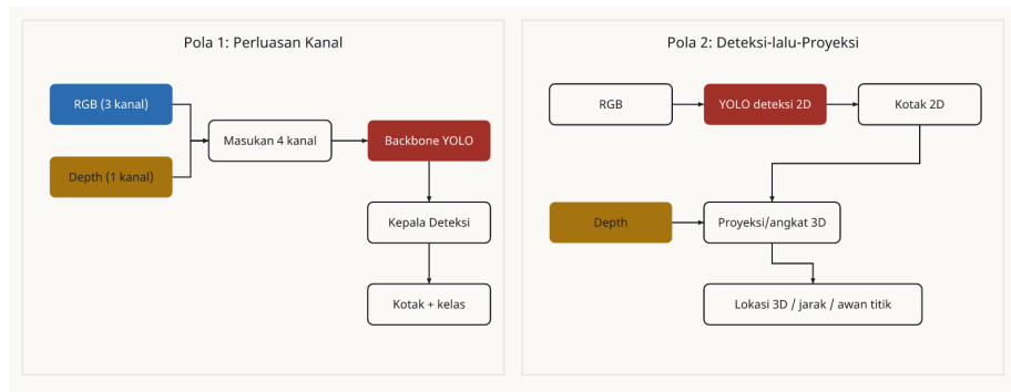
Gambar 6: Dua pola integrasi YOLO+RGB-D. Kiri: perluasan kanal masukan (fusi awal). Kanan: deteksi-lalu-proyeksi (kedalaman dipakai pascadeteksi).
