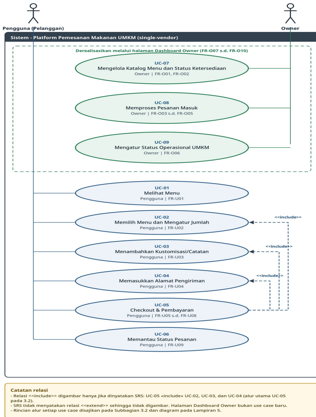
Gambar 1. Use Case Diagram Platform Pemesanan Makanan UMKM (UC-01 s.d. UC-09)
