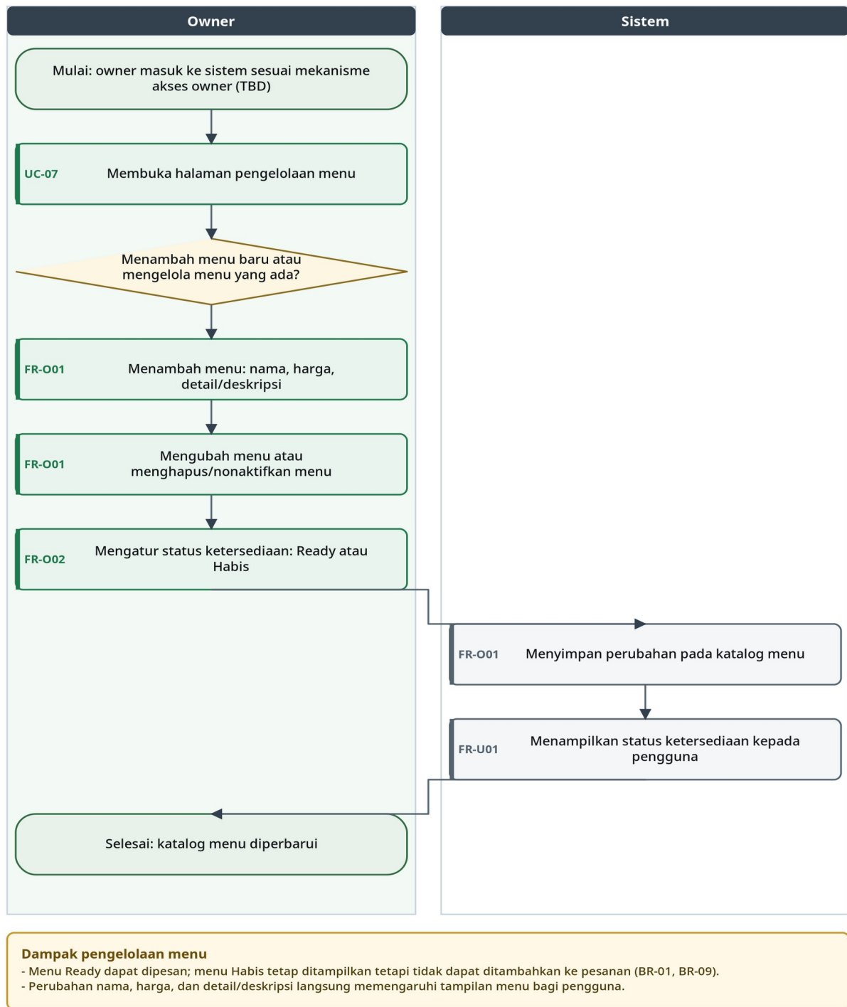
Gambar 3. Workflow Owner UC-07 - Mengelola Katalog Menu dan Status Ketersediaan
