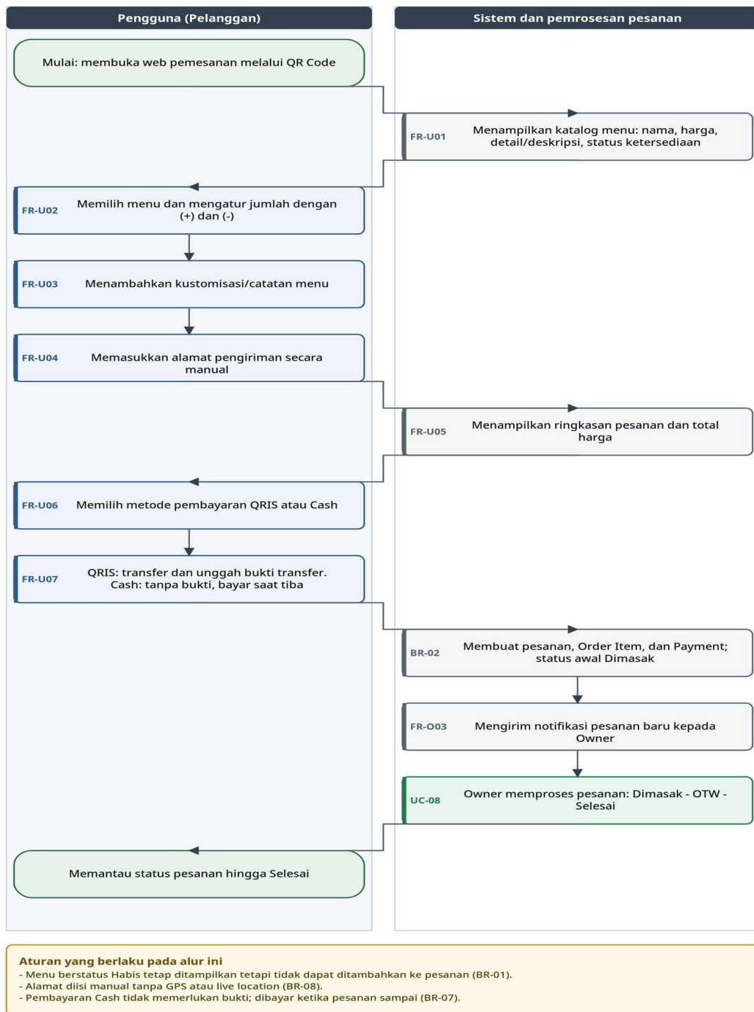
Gambar 2. Workflow Pemesanan Pelanggan (UC-01 s.d. UC-06)
