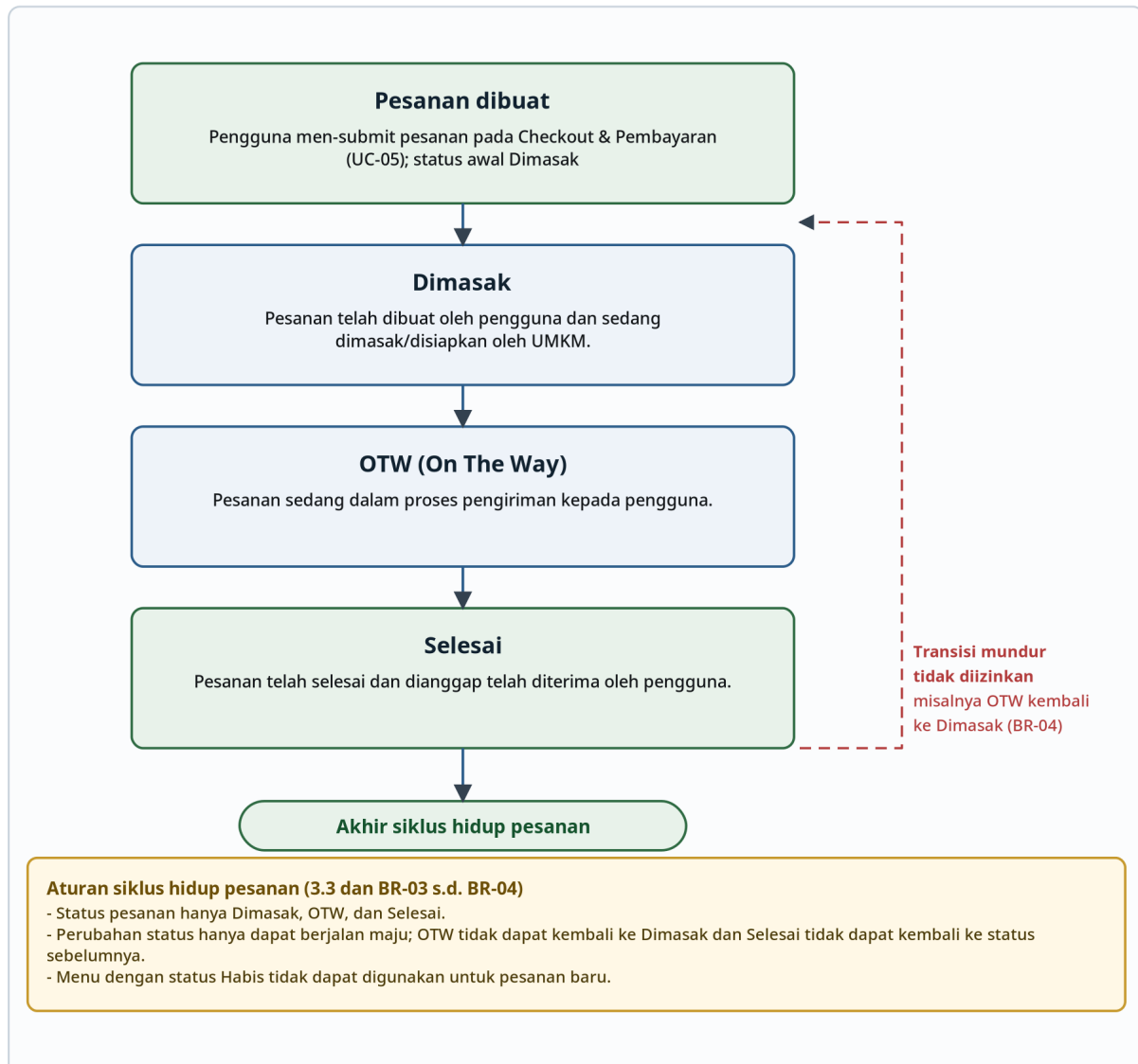
Gambar 7. Siklus Hidup Pesanan (Dimasak - OTW - Selesai)
