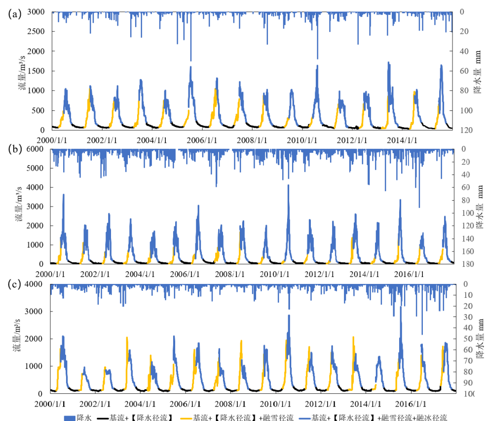
图 2.11 Gilgit(a)、Shyok(b)和 Kharmonig(c)流域逐日降水主导流量过程解析结果
