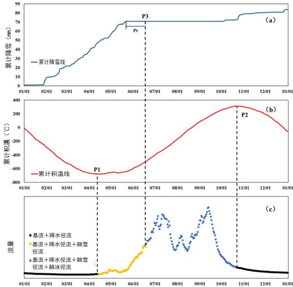
图 2.9 水文分区曲线示意图(a)累计逐日降雪曲线, (b)逐日积温曲线以及(c)水文分区曲线 (HPC)
