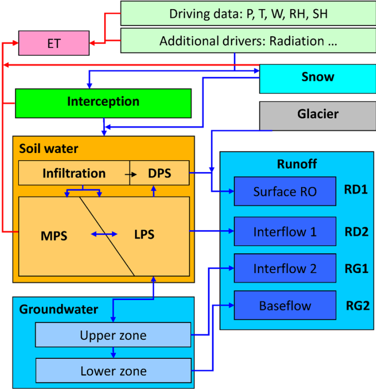
图 2.10 J2000 模型示意图
