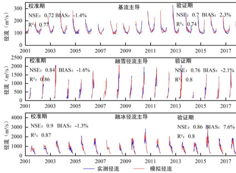
图 2.20 2001-2017 年 Khar Mong 流域基于 HPC 率定模型模拟径流与实测径流对比
