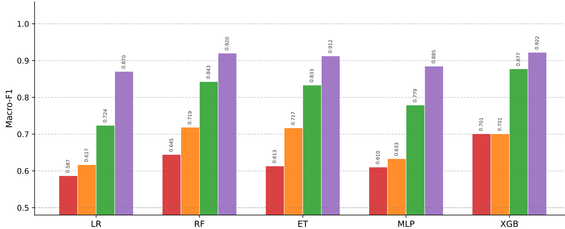
Tabular Models
