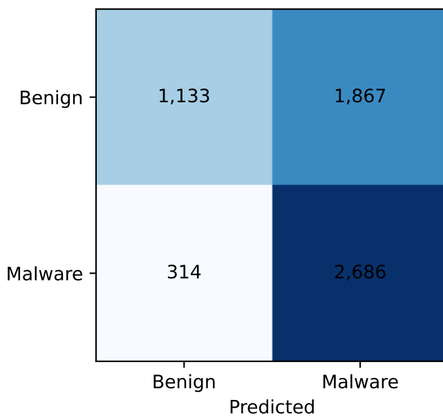
MLP
