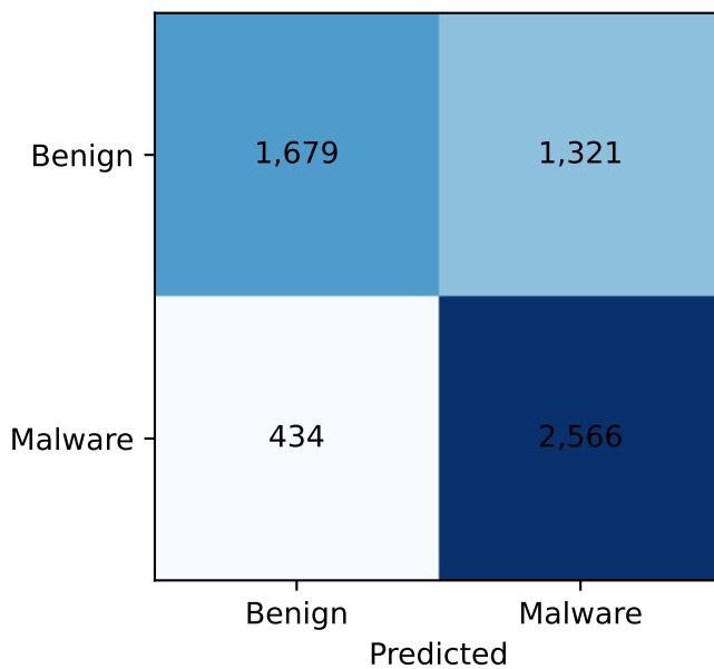
MLP
