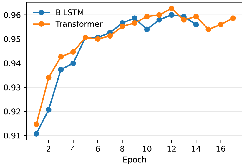
Validation Macro-F1
