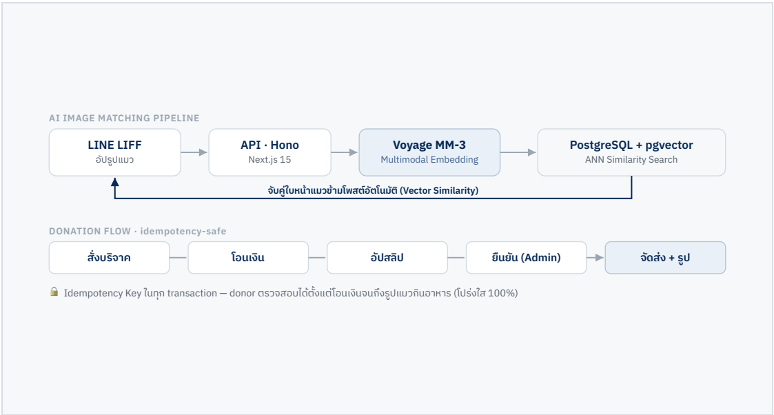
AI Vector Search Pipeline ของ MeawSook
