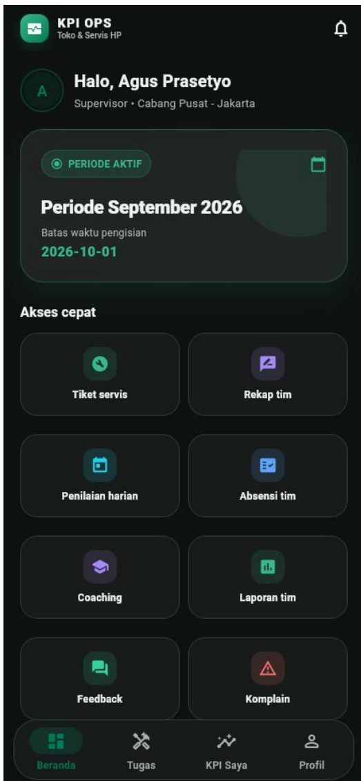
Gambar 25. Beranda Supervisor
