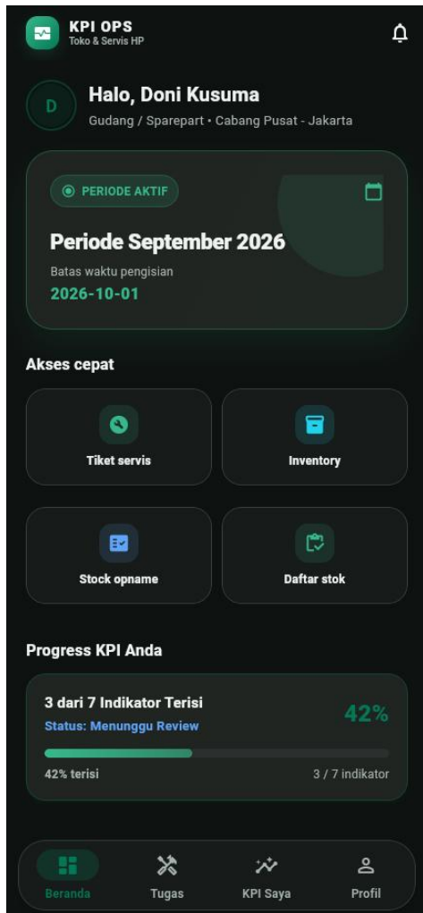
Gambar 20. Beranda Gudang
