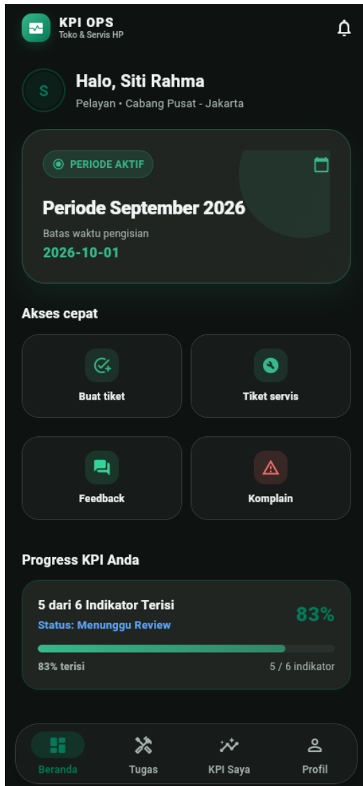
Gambar 12. Beranda Pelayan
