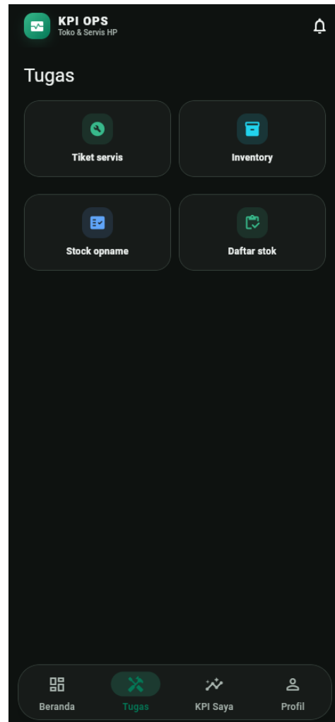
Gambar 21. Tugas Gudang
