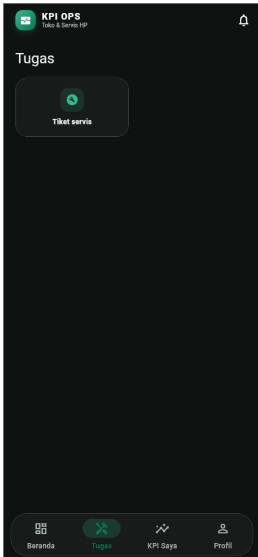
Gambar 15. Tugas Teknisi
