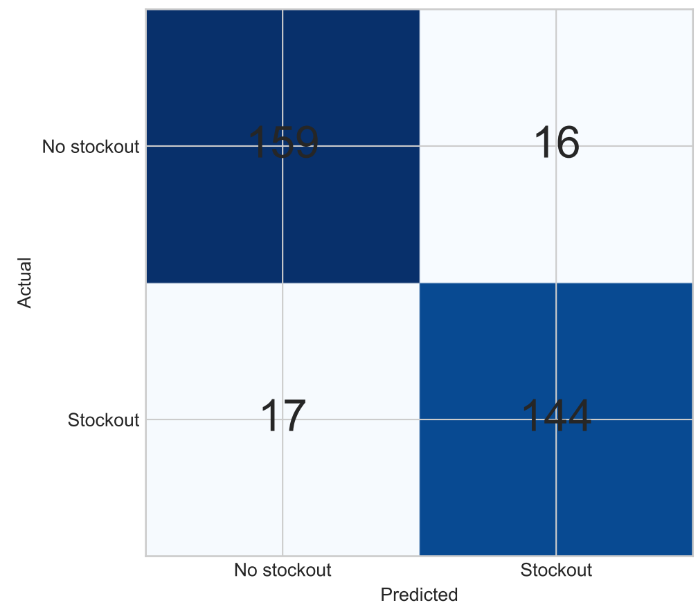
6h stockout confusion matrix · F1 0.897
