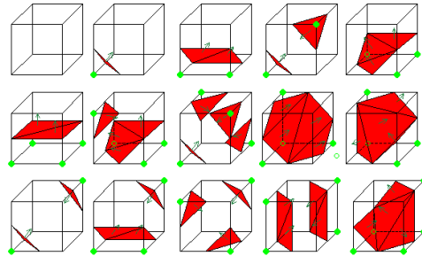
Figure 1: Configuración de Marching cubes
