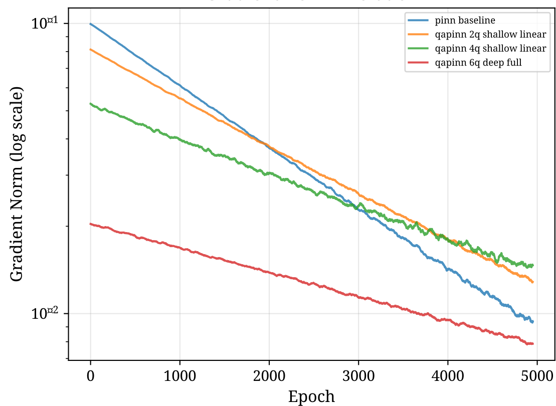
Gradient Norm Evolution
