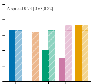
HaluEval-Sum
