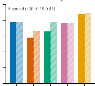
HaluEval-QA
