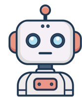
VLM
