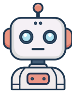
VLM
