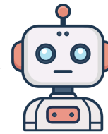
VLM
