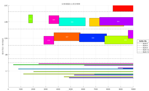
Matmul_Case0 分类型缓存占用甘特图
