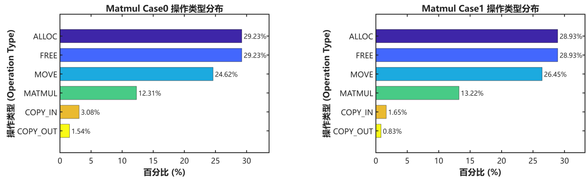
图 4.3 Matmul 系列数据集操作类型分布对比
