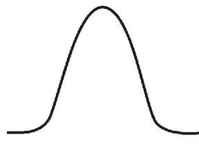
Curva leptocúrtica
