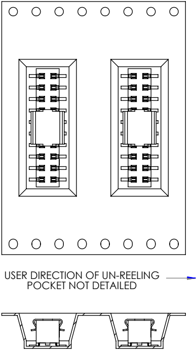
-DV-M STYLE SHOWN
