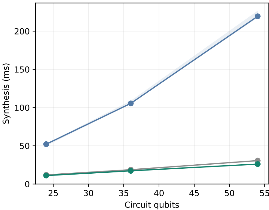
IQM R/CZ · Symbolic EfficientSU2
