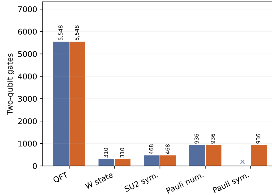
IBM SX/RZ/CZ · 156 qubits
