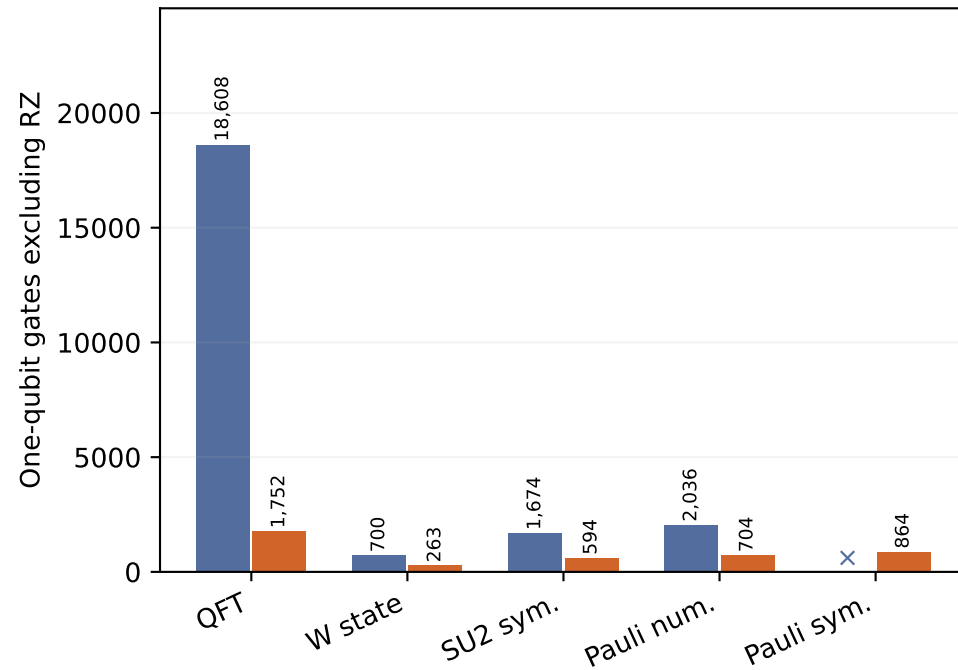
IQM R/CZ · 54 qubits
