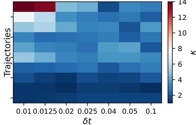
\kappa = N_B/N_A
