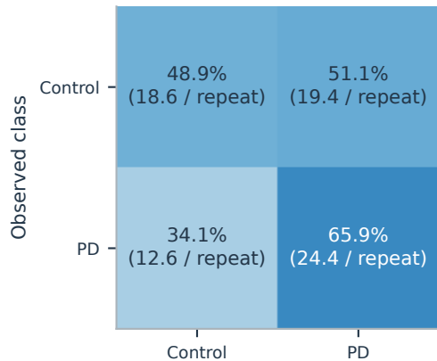
CNN
