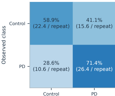
SVM
