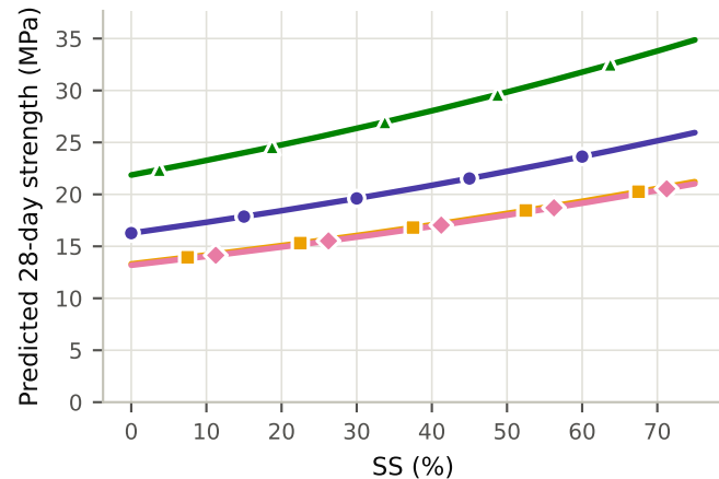
c 28 d — strength vs SS (RCF 30 %, A/B 0.45)
