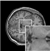
Input
