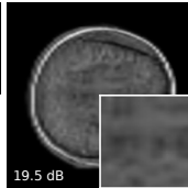
HCLD
