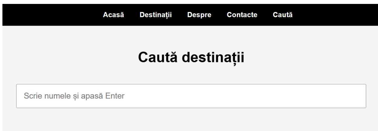
Fig. 3.6 - Secțiunea “Caută”
