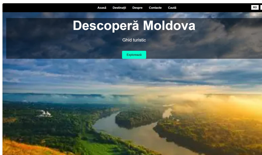
Fig. 3.2 - Pagina principală
