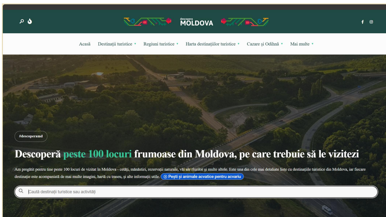
Figura 1.4 – Site similar
