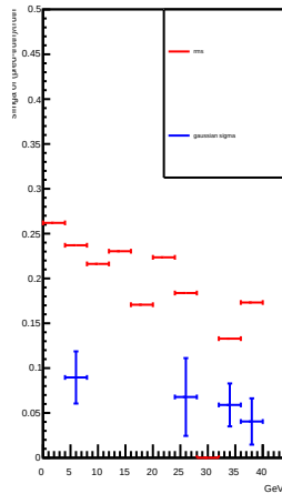
K0
