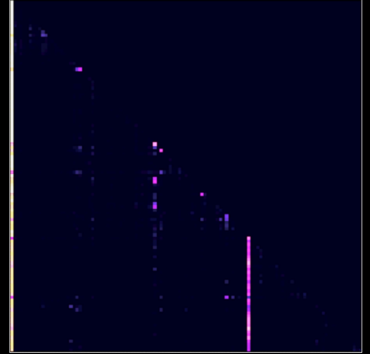
OATS
