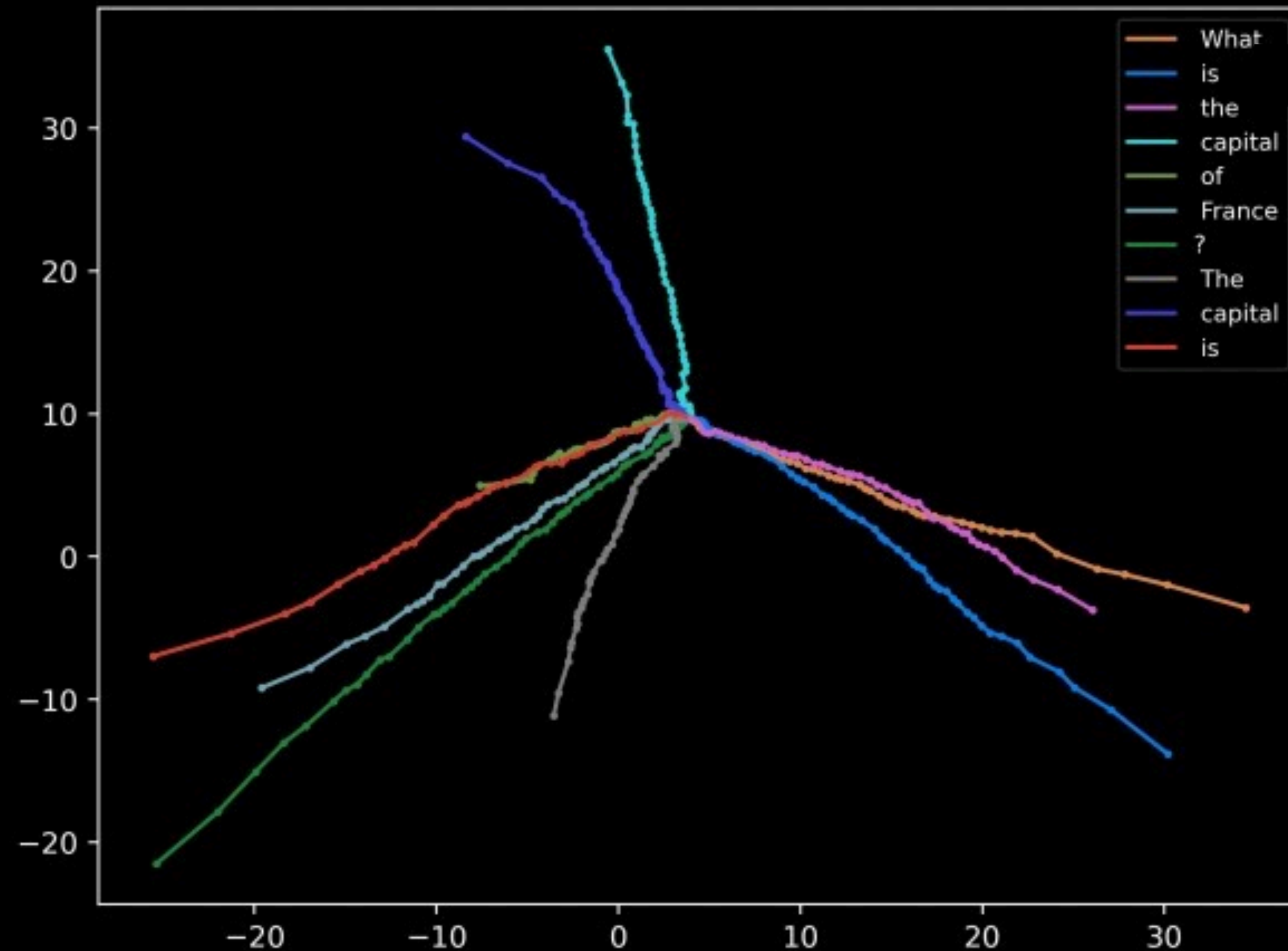
(a) Llama-3 70B
