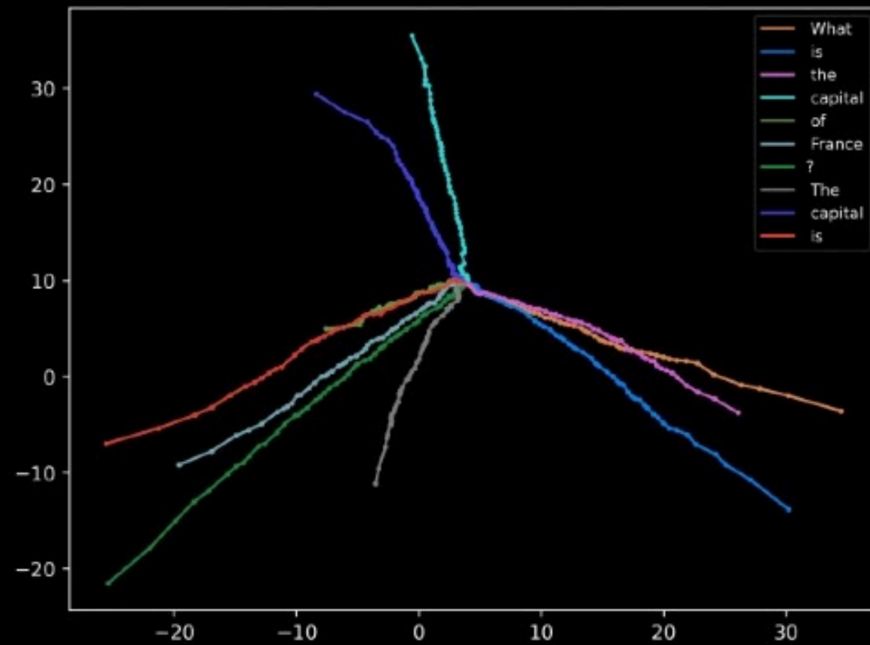
(a) Llama-3 70B
