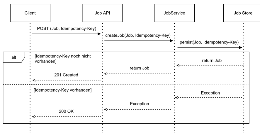
Abbildung 5.4: Ablauf der Jobannahme vom Eingang einer Anfrage über die Persistierung des Jobs bis zur Rückgabe einer Erfolgsnachricht an den Client inklusive Unterscheidung im Duplikatsfall des Idempotenz-Keys.
