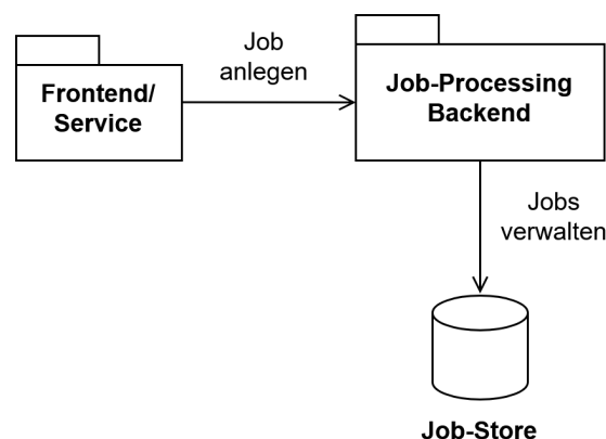
Abbildung 4.1: Systemkontext des entwickelten Background-Job-Processing-Systems: Clients übergeben Aufträge über die REST-Schnittstelle an das Backend, das diese persistent im Job-Store speichert. Anschließend werden die Jobs vom Backend asynchron verarbeitet.
