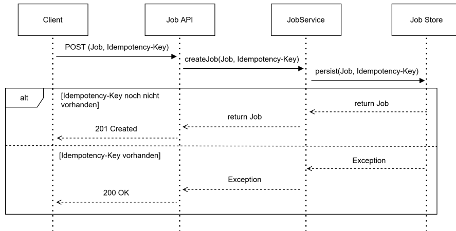
Abbildung 5.4: Ablauf der Jobannahme vom Eingang einer Anfrage über die Persistierung des Jobs bis zur Rückgabe einer Erfolgsmeldung an den Client inklusive Unterscheidung im Duplikatsfall des Idempotenz-Keys.
