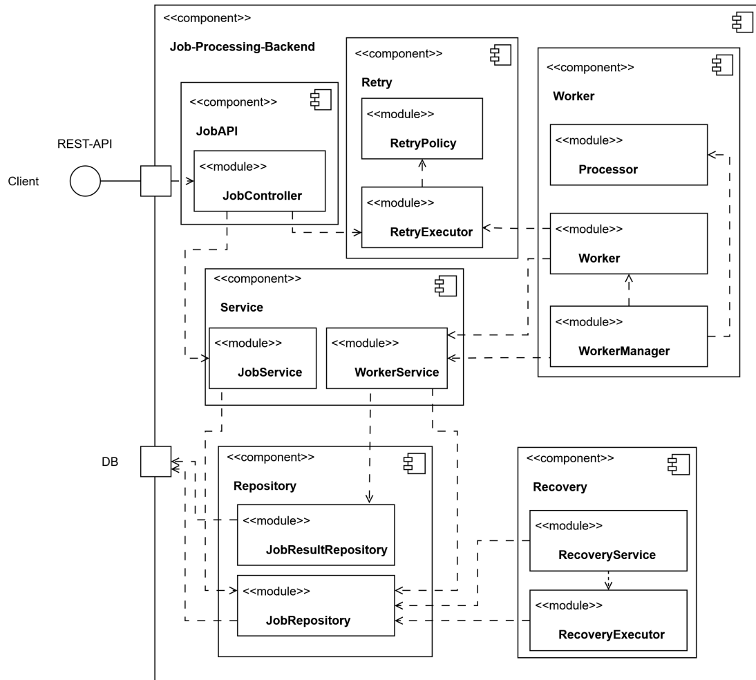
Abbildung A.1: Detaillierte Bausteinsicht des Job-Processing Backends mit Innensicht und Abhängigkeiten der unterschiedlichen Komponenten
