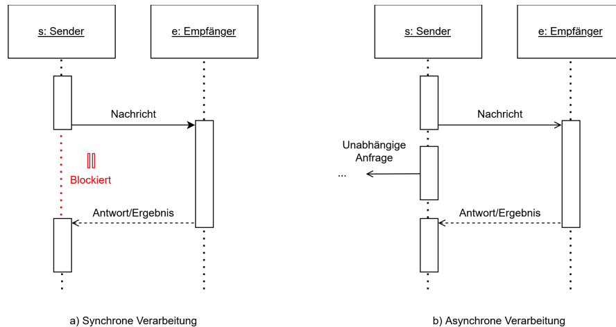
Abbildung 2.1: Vergleich der Kommunikationsmuster: (a) Bei der synchronen Verarbeitung blockiert der Aufrufer bis zum Erhalt der Antwort. (b) Die asynchrone Verarbeitung entkoppelt die Anfrage zeitlich von der Ergebnisantwort.
