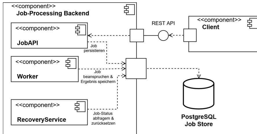
Abbildung 5.1: Bausteinsicht der Architektur des entwickelten Background-Job-Processing-Systems mit REST-Schnittstelle, Job-Store sowie der Worker-Komponente und dem Recovery-Service.
