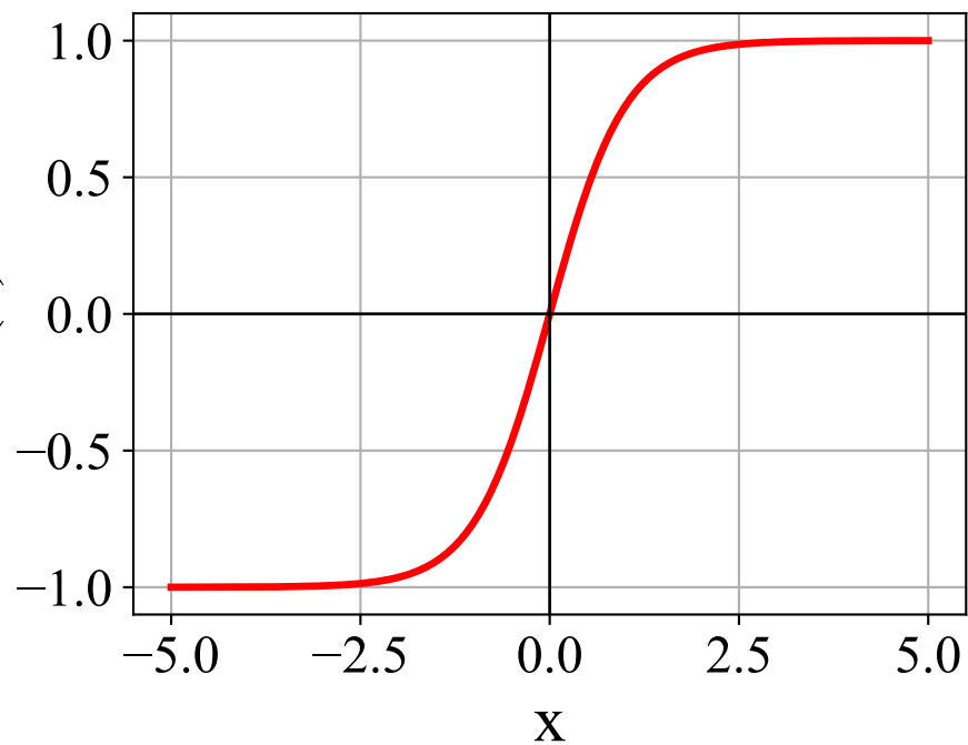
Tanh
