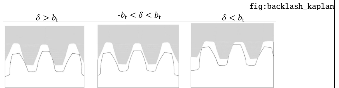
Figura 2.6 – Representação da folga de backlash
