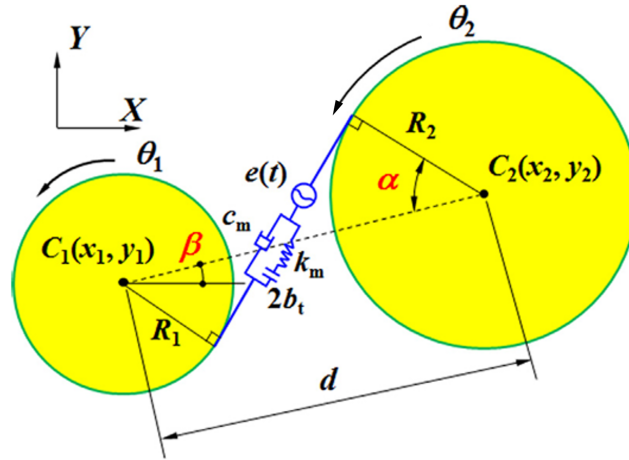
Figura 2.8 – Modelo de Par Engrenado
