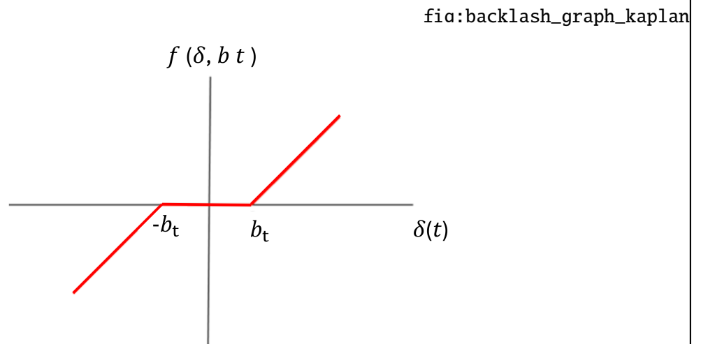
Figura 2.7 – Deformação da malha de engrenamento considerando a folga de backlash
