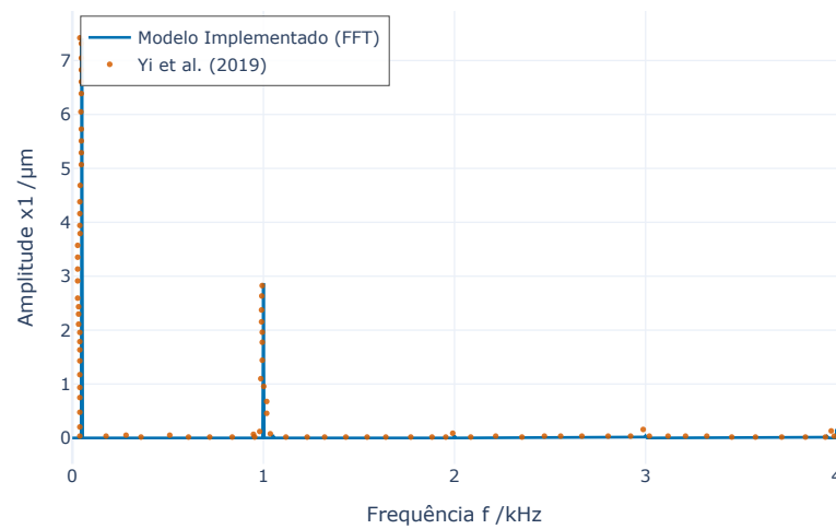
Fig 10(b) - Espectro FFT de x_1 a 3000 RPM
