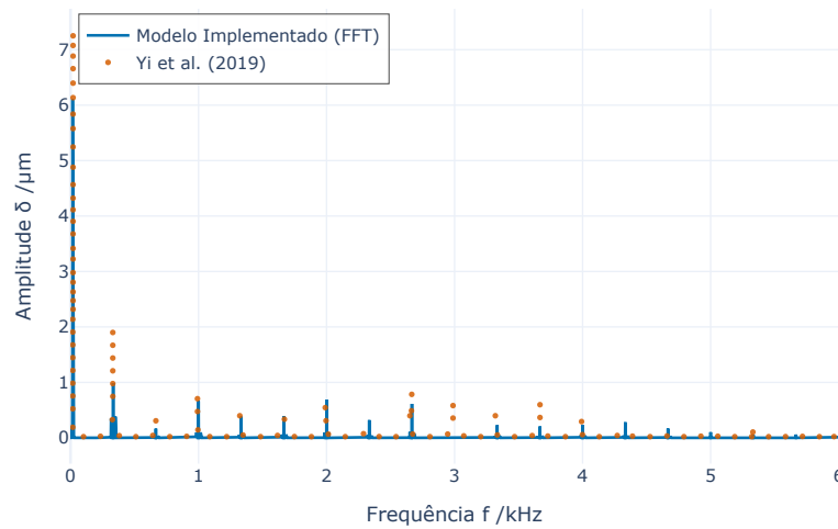
Fig 9(d) - Espectro FFT de \delta a 1000 RPM
