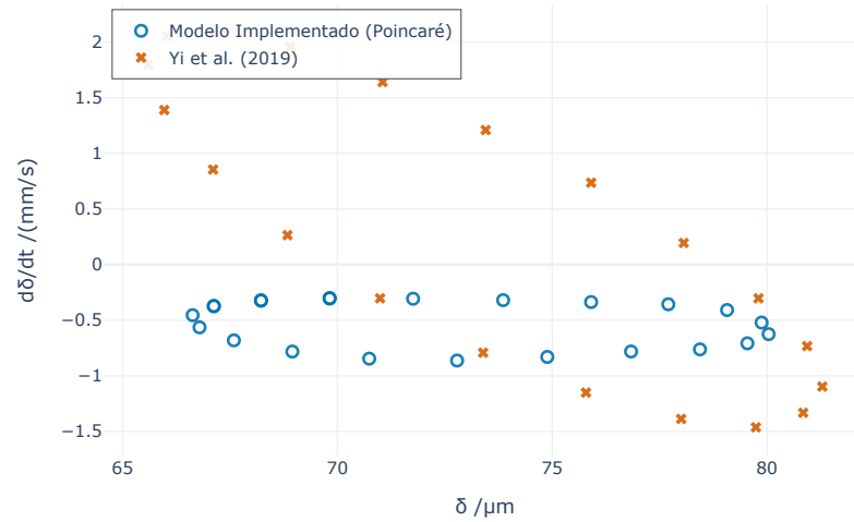
Fig 9(e) - Mapa de Poincaré de \delta a 1000 RPM
