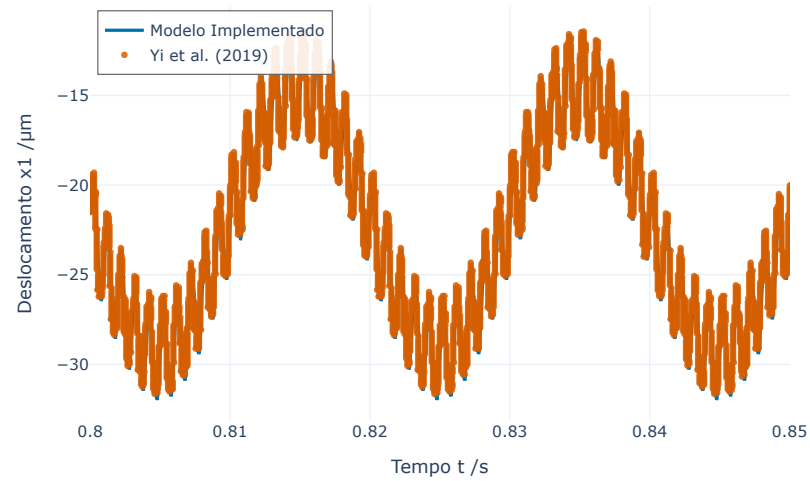
Fig 10(a) - Resposta de vibração x_1 a 3000 RPM
