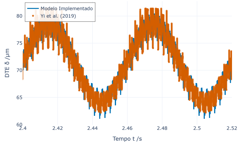
Fig 9(c) - Resposta de vibração \delta (DTE) a 1000 RPM
