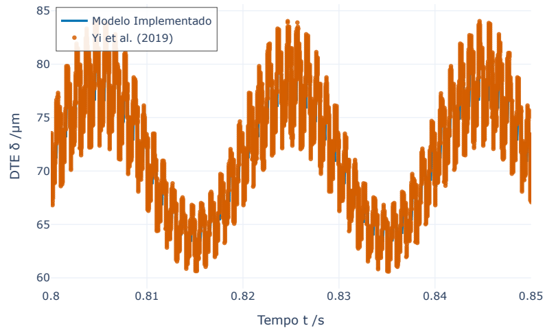
Fig 10(c) - Resposta de vibração \delta (DTE) a 3000 RPM
