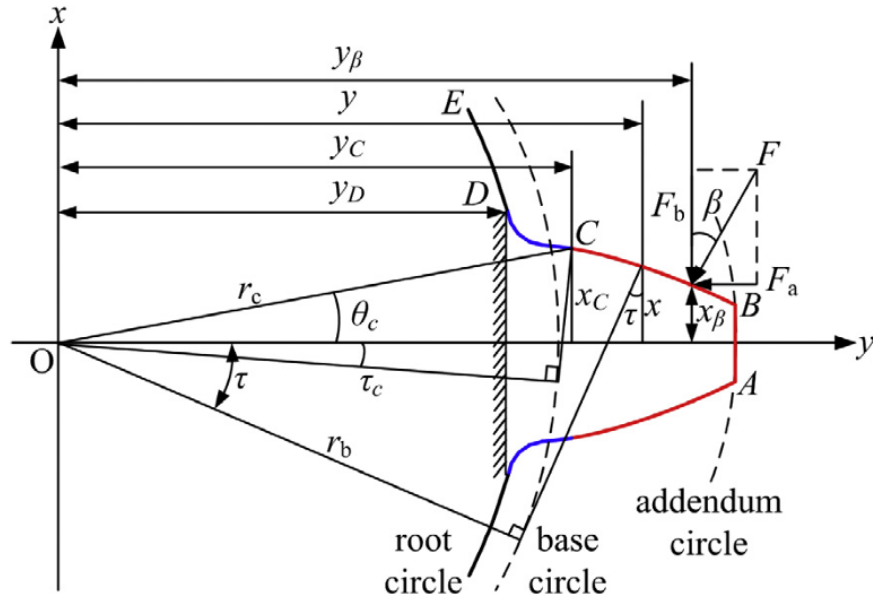
Figura 2.17 – Modelo geométrico do perfil do dente da engrenagem
