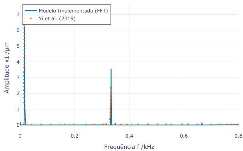
Fig 9(b) - Espectro FFT de x_1 a 1000 RPM
