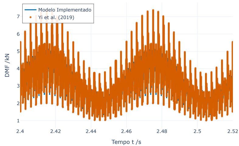
Fig 9(f) - Resposta no tempo da DMF a 1000 RPM
