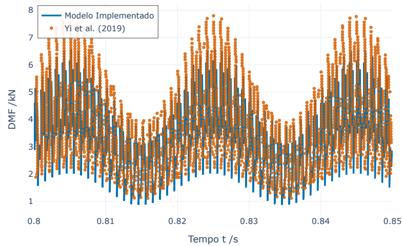
Fig 10(f) - Resposta no tempo da DMF a 3000 RPM
