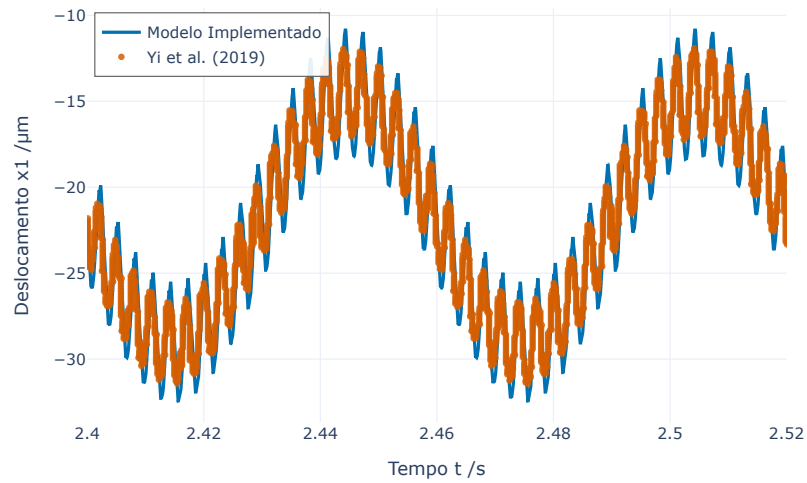
Fig 9(a) - Resposta de vibração x1 a 1000 RPM
