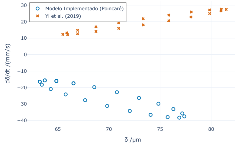
Fig 10(e) - Mapa de Poincaré de \delta a 3000 RPM
