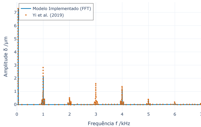
Fig 10(d) - Espectro FFT de \delta a 3000 RPM
