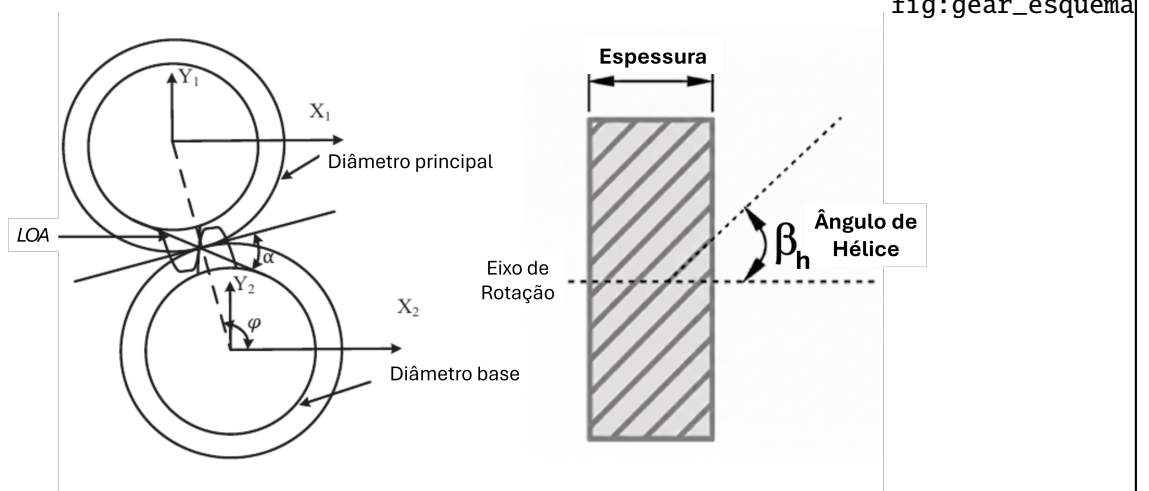
Figura 2.4 – Representação esquemática de uma engrenagem.
