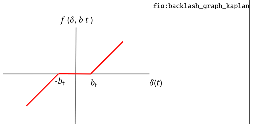
Figura 2.17 – Deformação da malha de engrenamento considerando a folga de backlash
