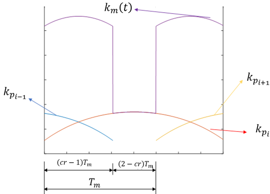
Figura 2.14 – Perfil de rigidez do engrenamento correlacionado com razão de contato
