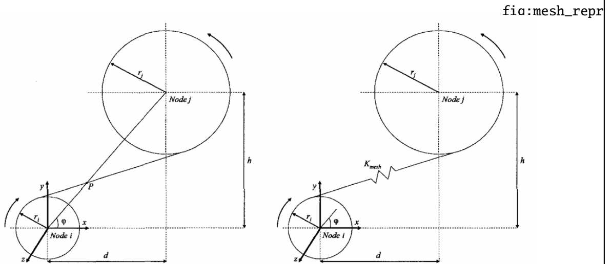
Figura 2.9 – Reapresentação do Engrenamento
