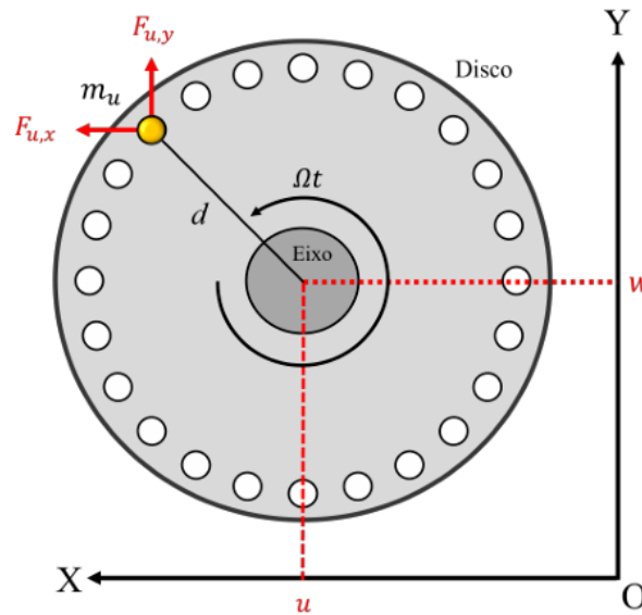
Figura 2.4 – Representação esquemática do desbalanceamento.
