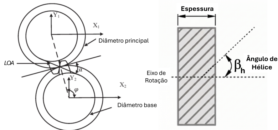
Figura 2.8 – Representação esquemática de uma engrenagem.
