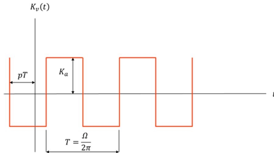
Figura 2.12 – Perfil de rigidez do engrenamento correlacionado com razão de contato
