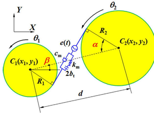
Figura 2.18 – Modelo de Par Engrenado
