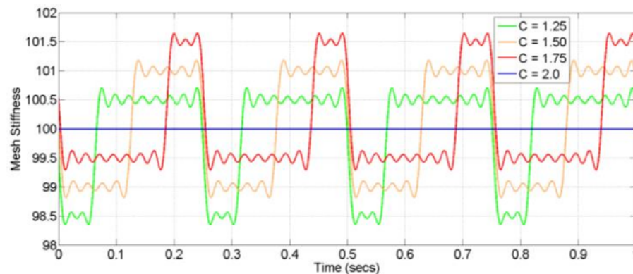
Figura 2.13 – Perfil de rigidez do engrenamento correlacionado com razão de contato
