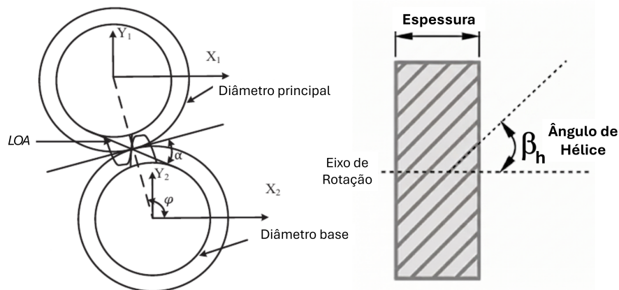
Figura 2.7 – Representação esquemática de uma engrenagem.
