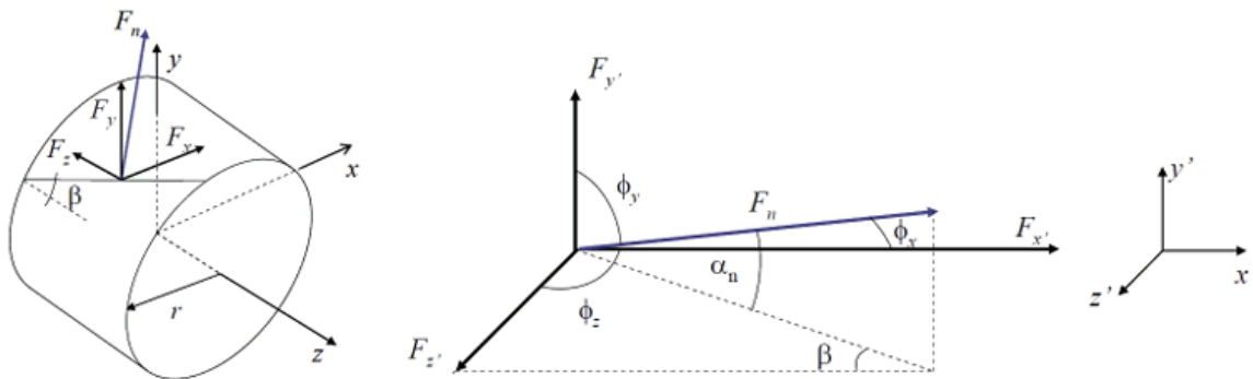
Figura 2.10 – Decomposição das forças no ponto de contato das engrenagens.
