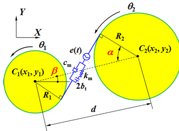
Figura 2.17 – Modelo de Par Engrenado
