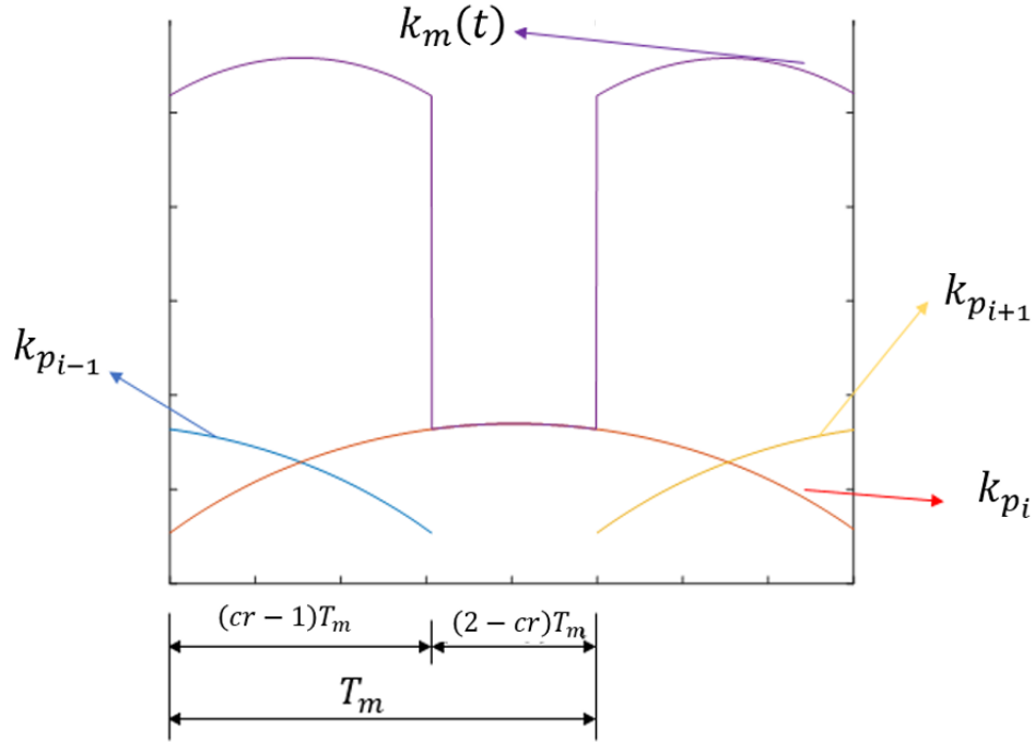
Figura 2.13 – Perfil de rigidez do engrenamento correlacionado com razão de contato
