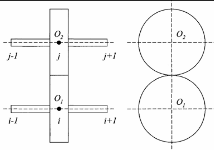
Figura 2.6 – Representação do par engrenado em elementos finitos (STRINGER, 2008) fig:gear_repr
