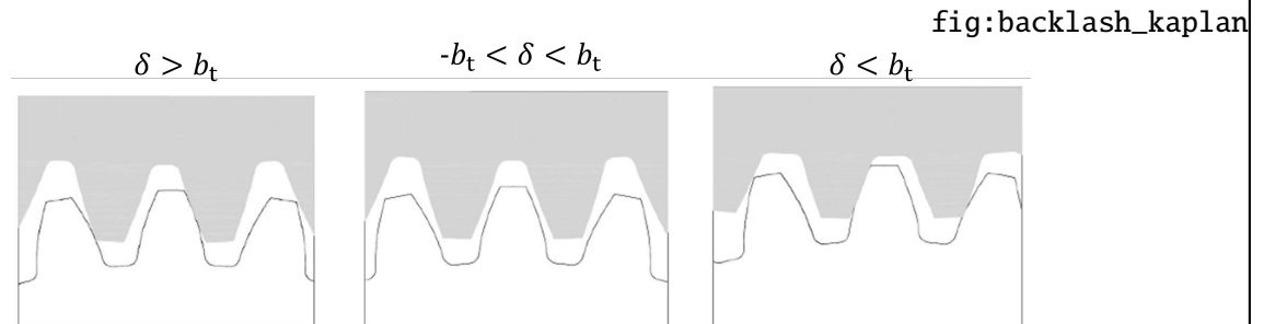
Figura 2.12 – Representação da folga de backlash
