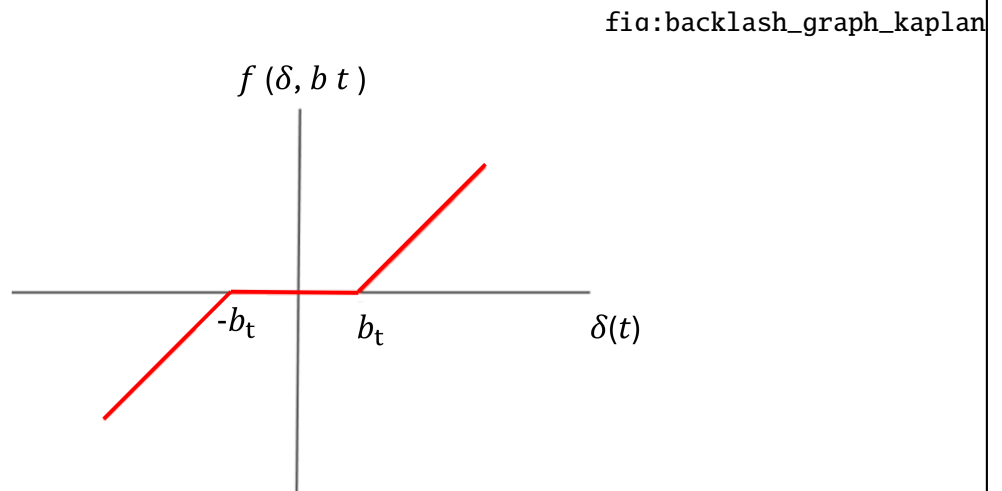
Figura 2.12 – Deformação da malha de engrenamento considerando a folga de backlash
