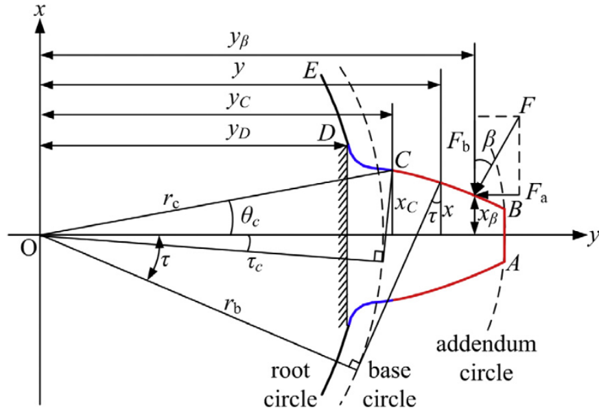
Figura 2.10 – Modelo geométrico do perfil do dente da engrenagem
