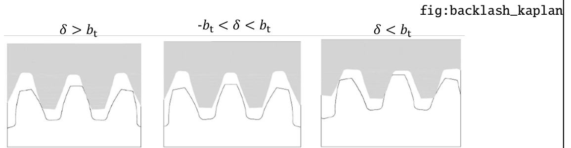
Figura 2.11 – Representação da folga de backlash
