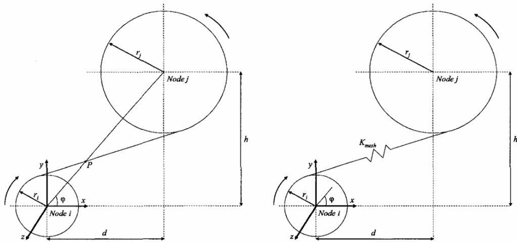
Figura 2.4 – Reapresentação do Engrenamento
