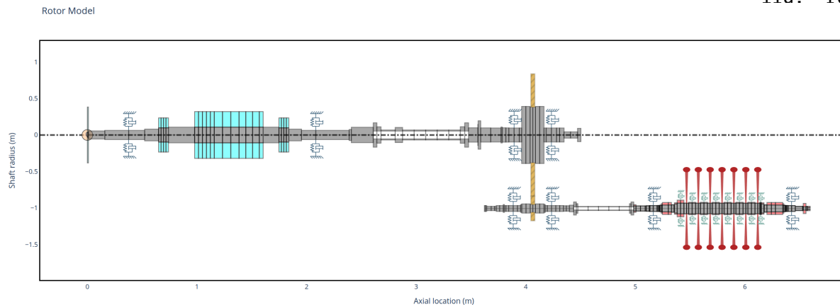
Figura 2.2 – Exemplo de rotores engrenados no ROSS
