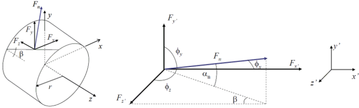
Figura 2.6 – Decomposição das forças no ponto de contato das engrenagens.
