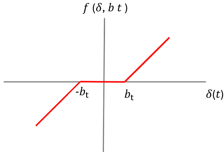
Figura 2.3 – Deformação da malha de engrenamento considerando a folga de backlash
